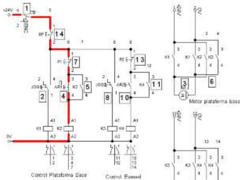
Figura 2.12 Arranque por pulsador
