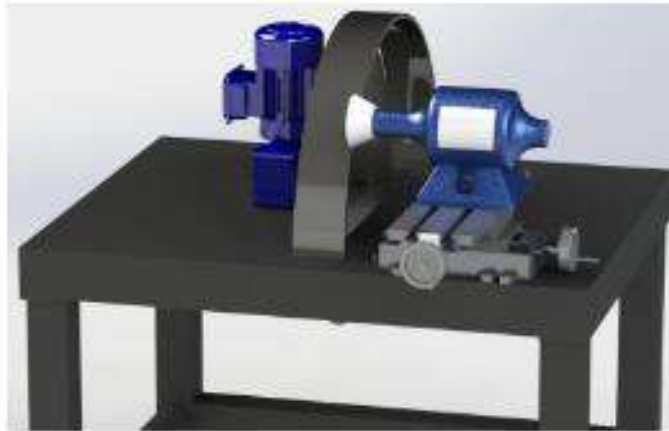
Figura 3.3 Máquina afiladora (vista lateral)
