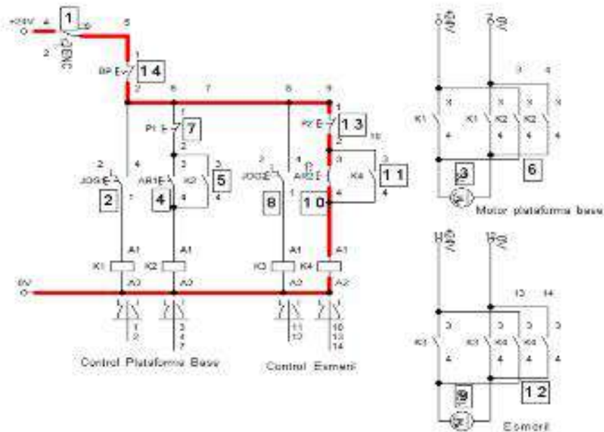
Figura 2.21 Trabajo continuo
