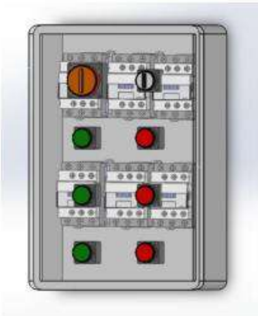
Figura 3.4 Propuesta del tablero de control
