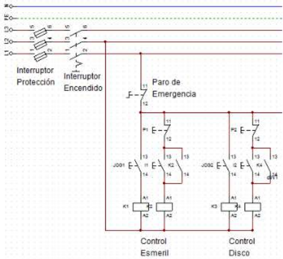
Figura 2.28 Interruptores de encendido y control por jogeo y paro-arranque
