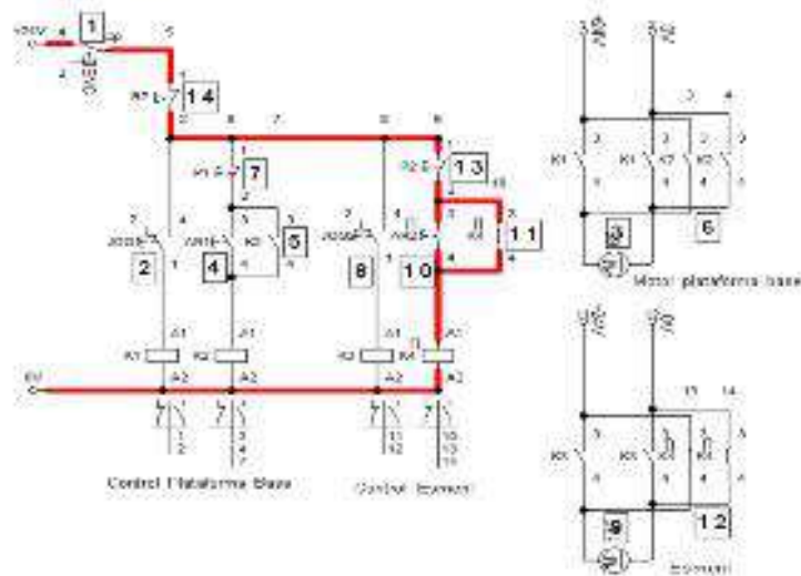
Figura 2.22 Contactor energizado
