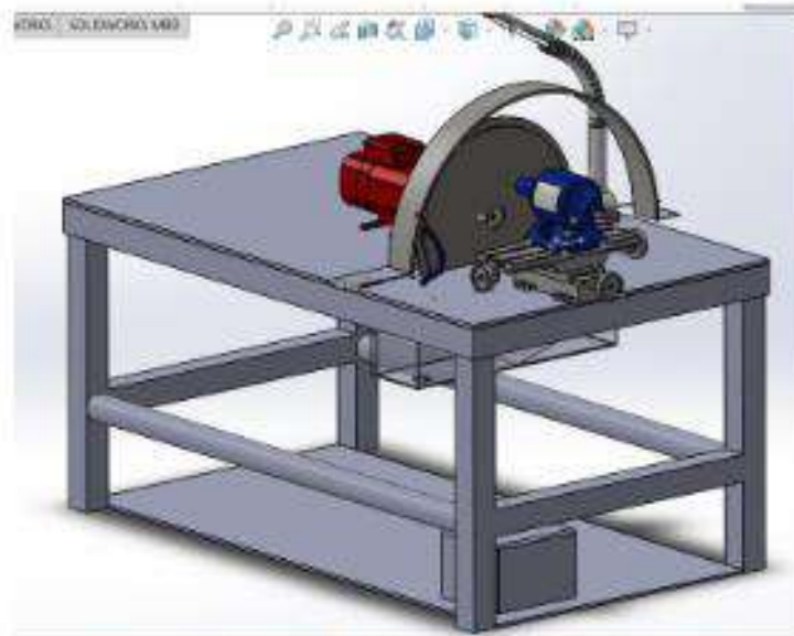
Figura 2.2 Afiladora de sierra circular en posición vertical
